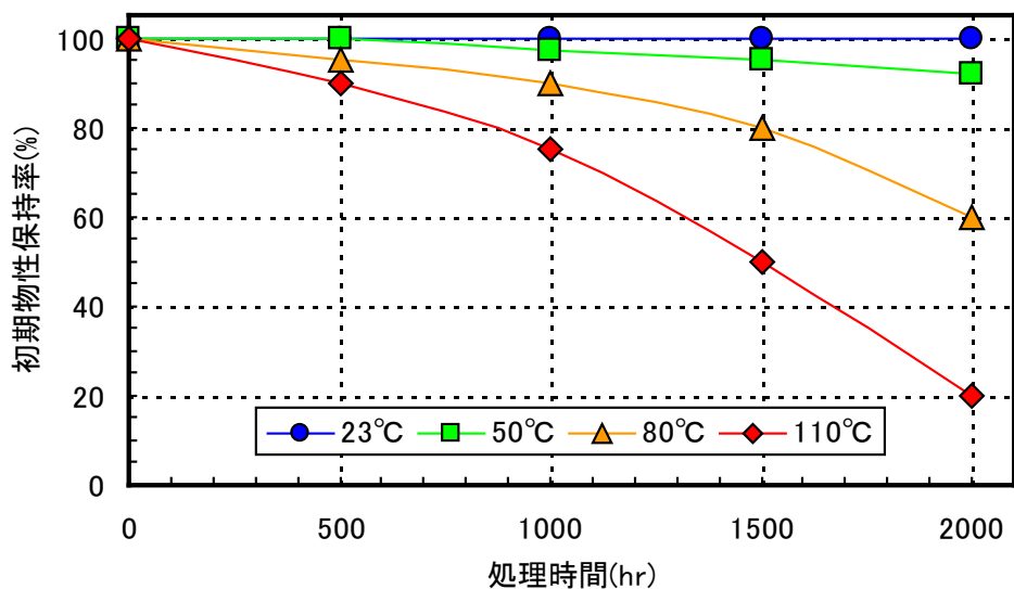
耐久性(耐熱性)試験結果例
