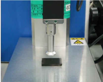
デュロメータ硬さ計測定部
