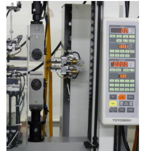
<引張試験機>
